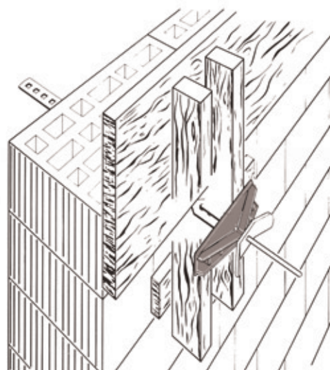
Stirnschalungsschraube BS 20 zum einfachen Abschalen der Decke oder Weiterschalen mit Kanthölzern
