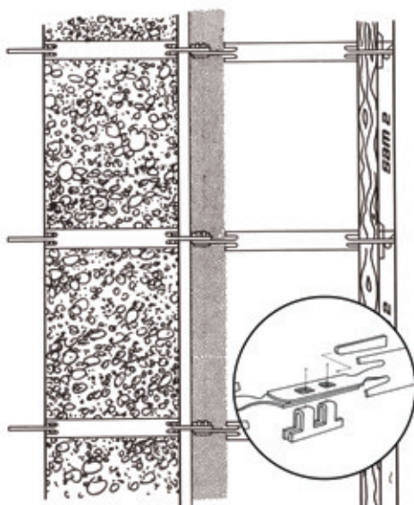
Doppelwand Verbindungsstück zum Verbinden von Abstandhaltern bei Doppelmauern (Isolierung)
