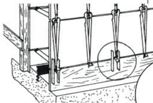
Holzausgleich ohne Zersägen von Schalungsplatten
