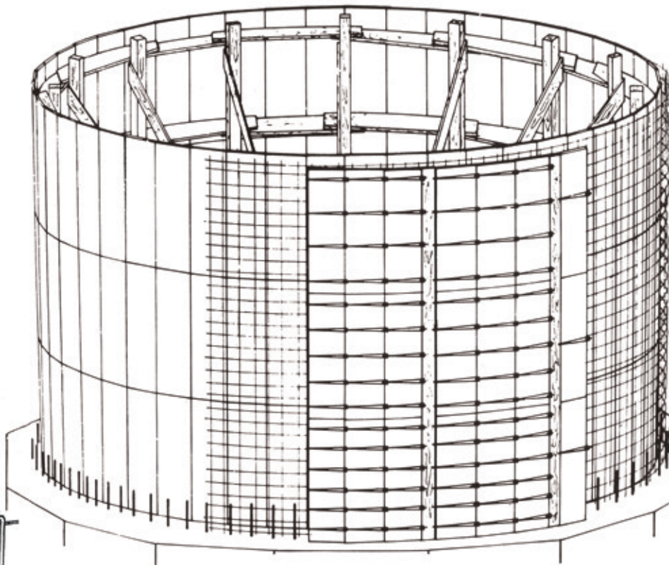
SAM Rundschalung
