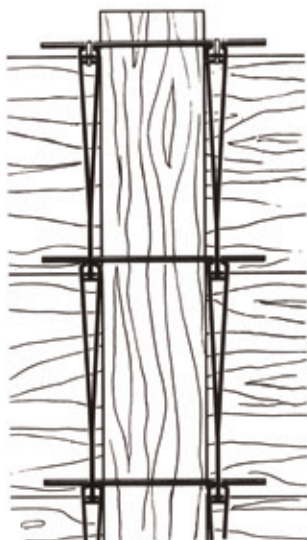
Holzausgleich ohne Zersägen von Schalungsplatten
